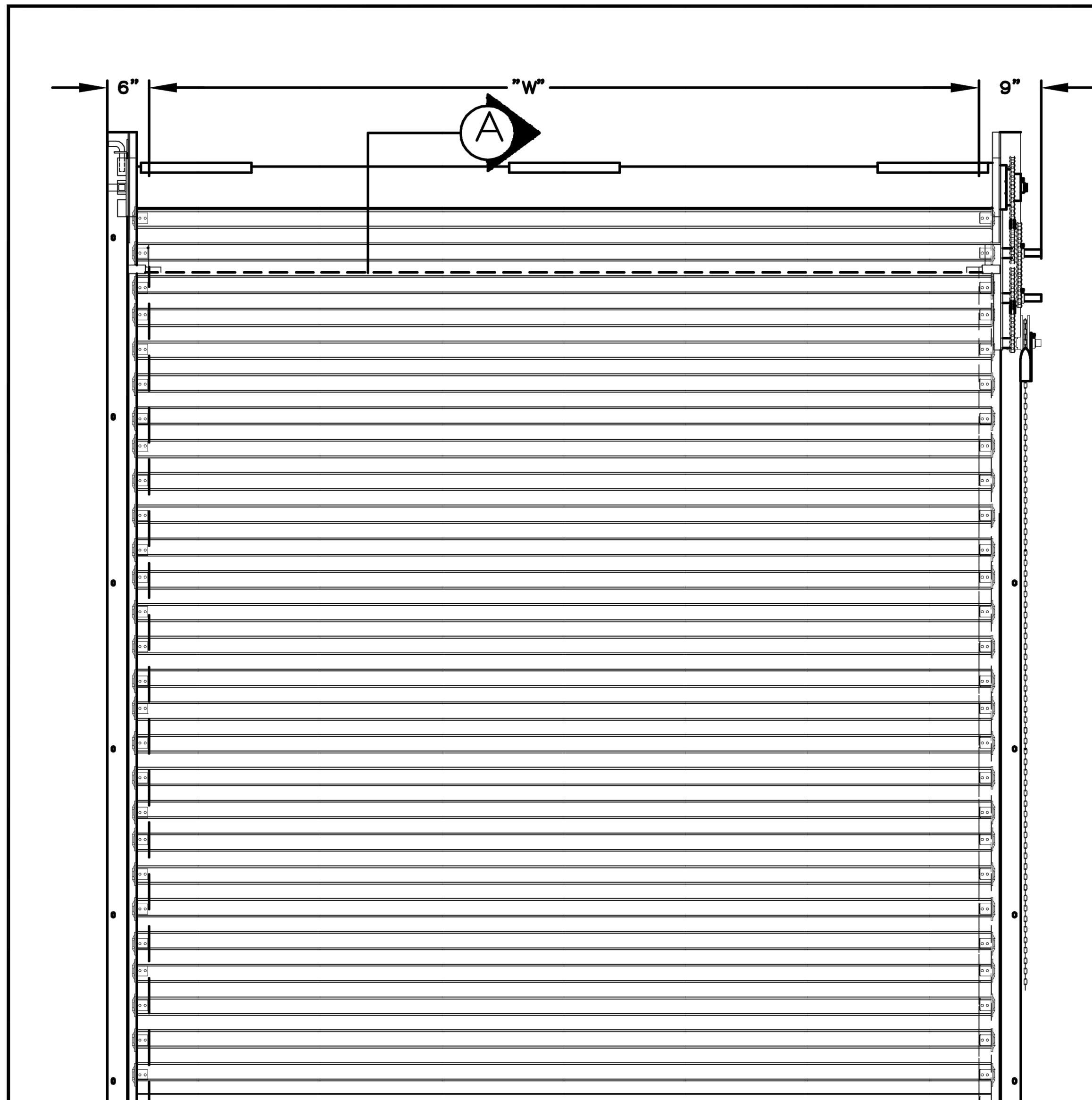
ELEVATION
