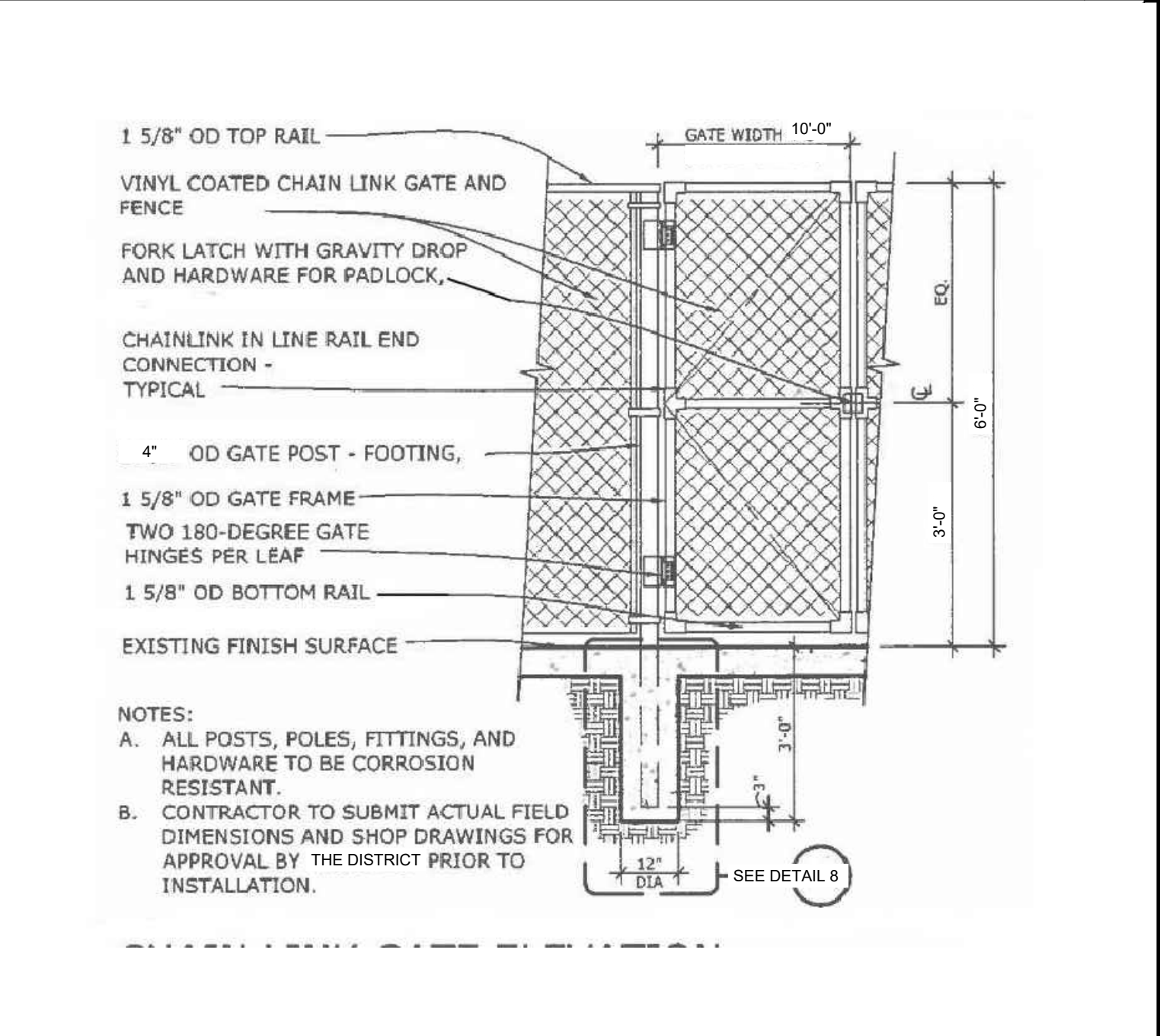
CHAIN LINK FENCE DETAILS SCALE: N.T.S. 3
