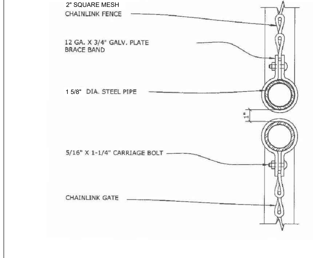
CHAINLINK GATE HEAD SCALE: 3"=1'-0" 4
